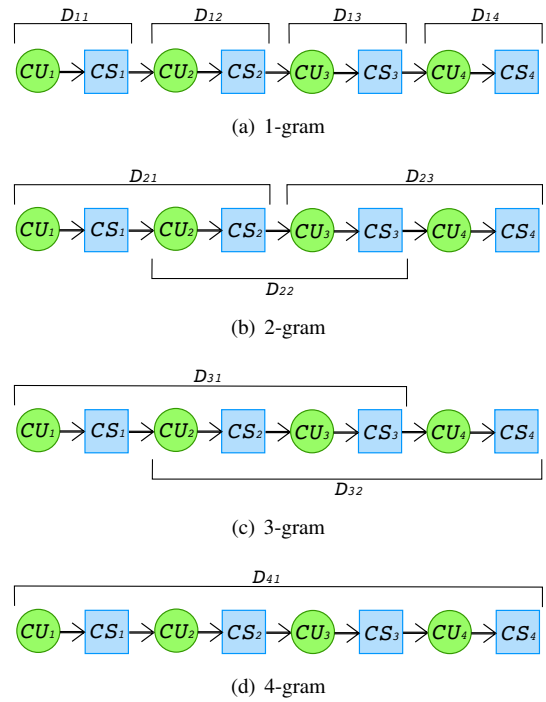
図2 ACNによる分割例 (M=4 の場合)
