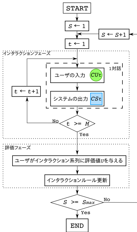
図1 インタラクションモデル
